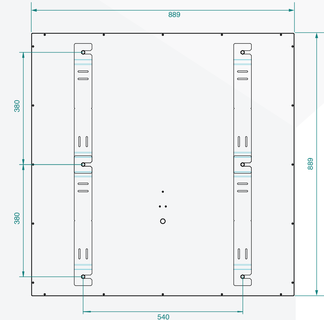
Backside Leranti® Easy 90x90
